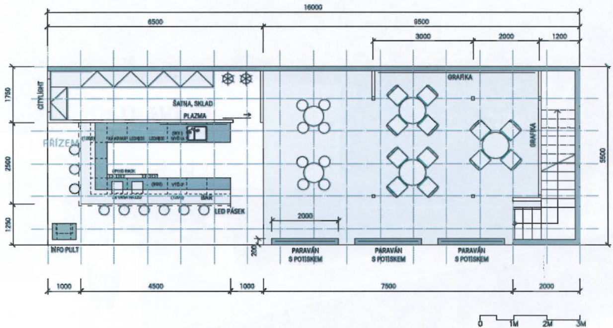
PŮDORYS 1NP
